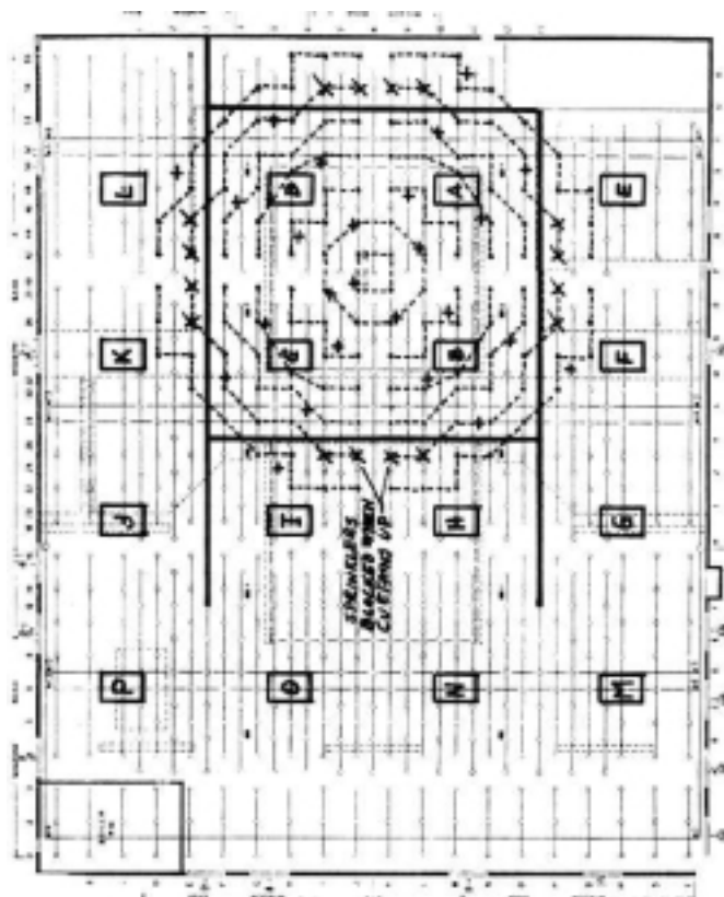
Figur 3 Bilden visar placering av sprinkler, brandventilatorer och röskärmar i de modellskaletesterna som genomfördes av FMRC år 1974.
