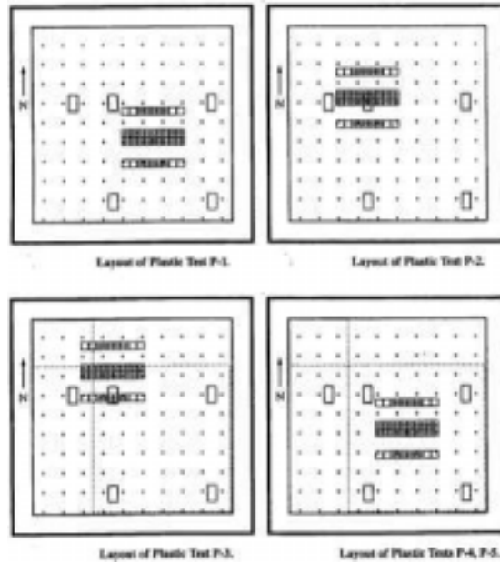
Figur 7 Layout för försöken med FMRCs "standard plastic" gods.
